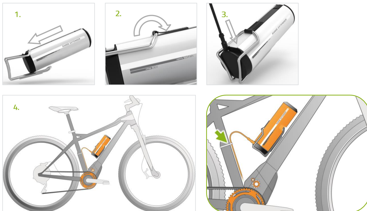
Abbildung 4: Montage mit Flaschenhalter
